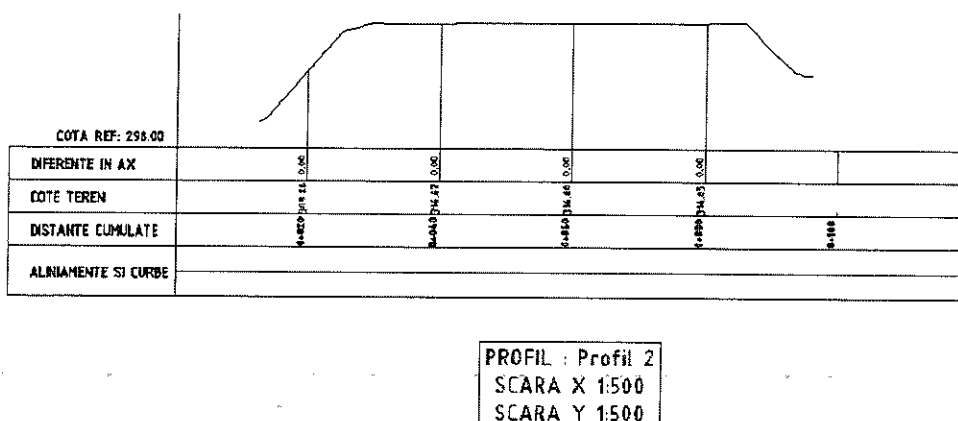
Fig. 6: Profilul transversal 2 – 2
