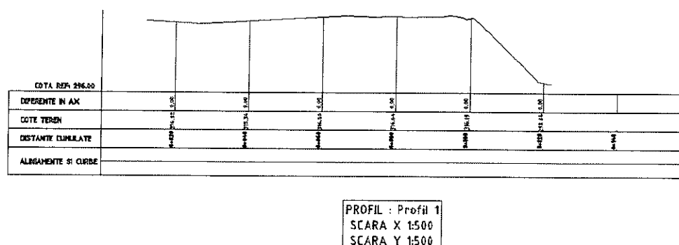
Fig. 5: Profilul transversal 1 – 1
