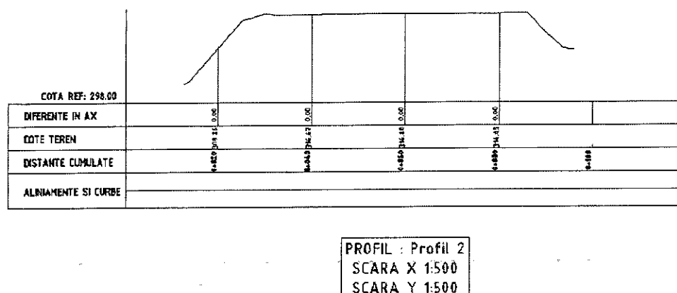
Fig. 6: Profilul transversal 2 – 2
